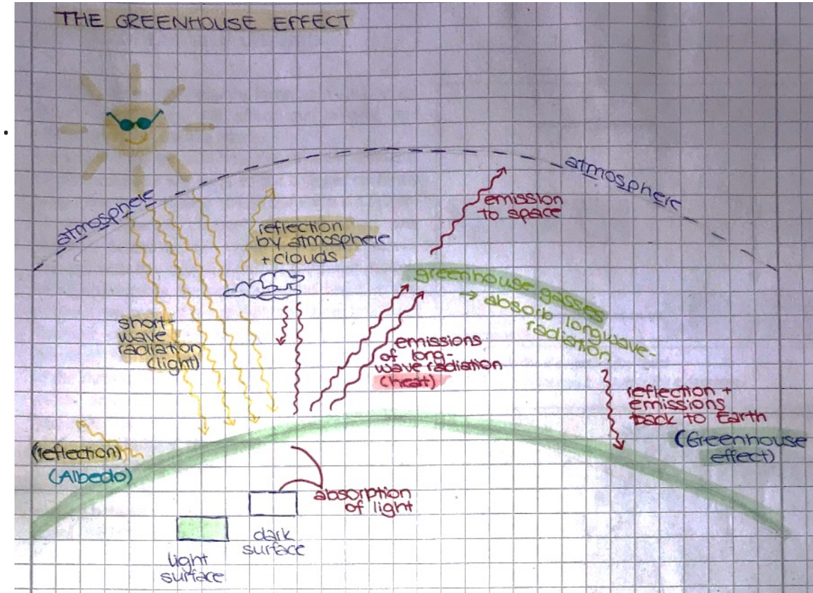
Schaubild zum Treibhauseffekt, Erdkunde Klasse 10
